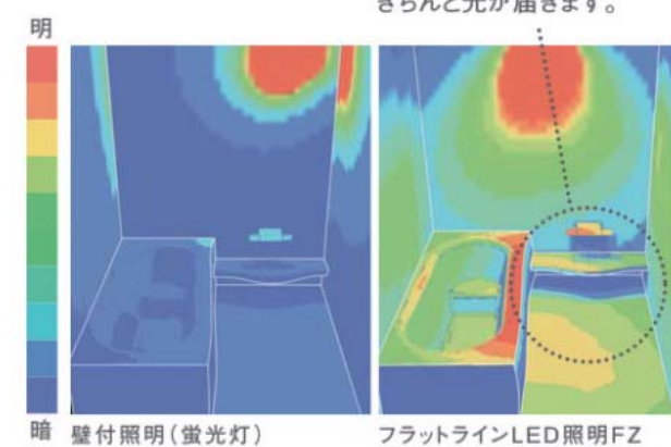
◎浴室内照度分布図
